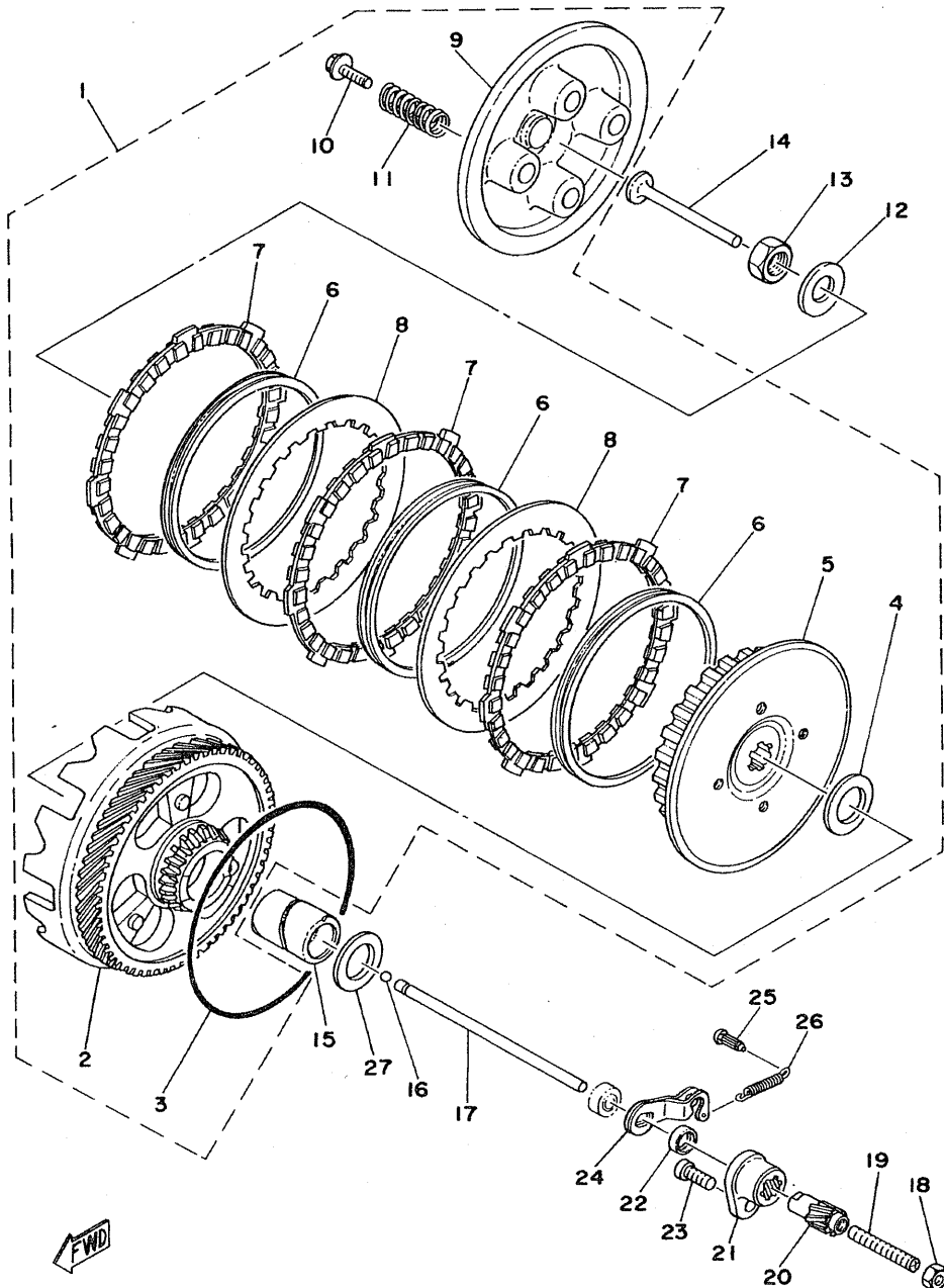
Fig. 4 CLUTCH
